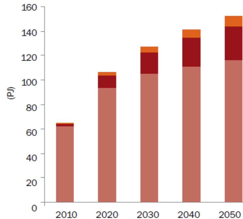
Graf 12: Potenciál výroby tepla z obnovitelných zdrojů
